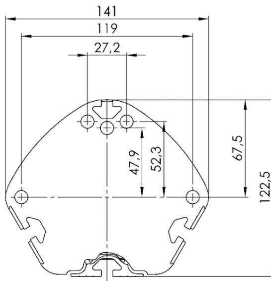
Strip ('Nutenstein') voor montage in buitenprofiel
