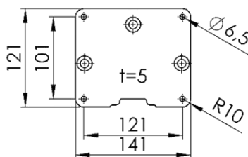
Montageplaat
