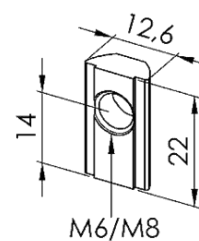
Strip ('Nutenstein') voor montage in buitenprofiel
